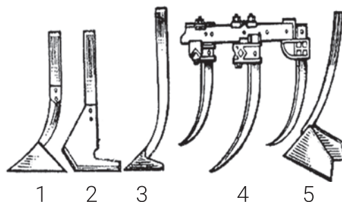
Рисунок 10. Рабочие узлы культиватора: 1 – режущая лапа; 2 – односторонняя режущая лапа; 3 – стреловидная лапа; 4 – лапа с пружиной; 5 – лапа с двусторонней режущей кромкой.
