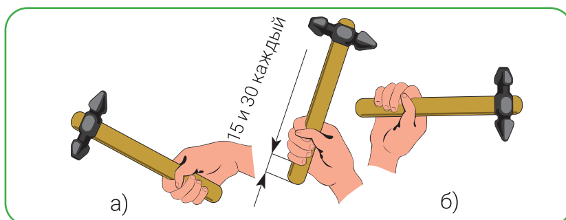
Рисунок 42. Виды хвата рук при работе молотком: а) с разжатыми пальцами; б) со сжатыми пальцами.
