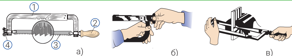
Рис 33. Регулировка полотна: а) полотно устанавливается в плоскости станины; б) натяжение полотна; в) полотно монтируется перпендикулярно плоскости каркаса.
