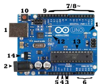
Рисунок 2. Устройство Arduino UNO
