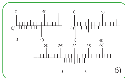
Рисунок 24. Штангенциркуль марки ШЦ-I:
