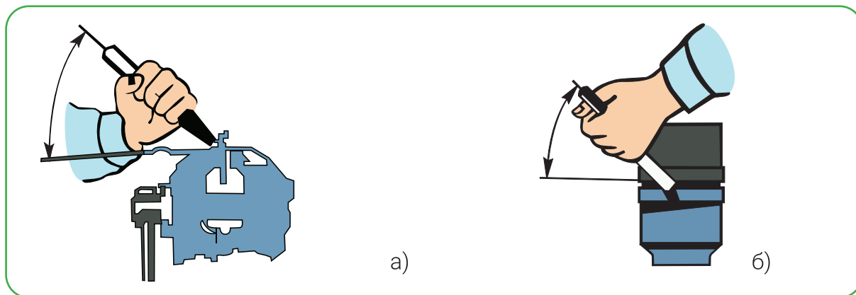
Рисунок 39. Схема установки зубила к обрабатываемой поверхности: а) угол рубки; б) угол наклона.
