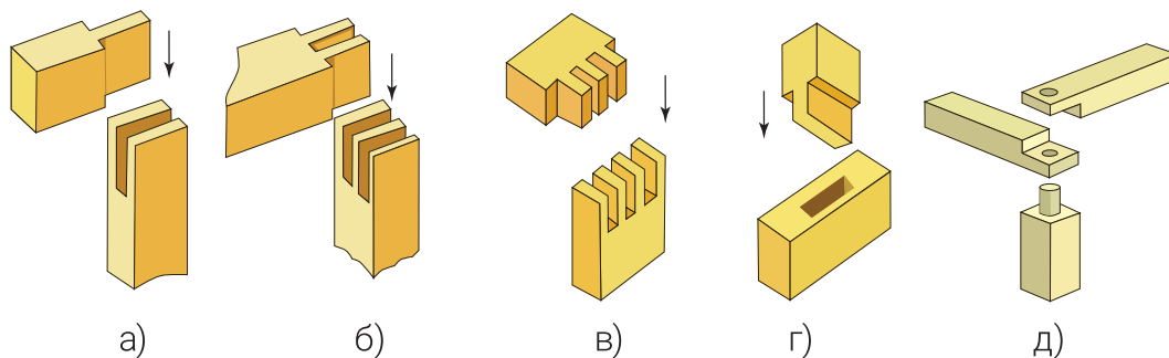
Рисунок 21. Способы столярных соединений: а) одинарный шип; б) двойной шип; в) тройной шип; г) с закрытым пазом; д) комплексное соединение.
