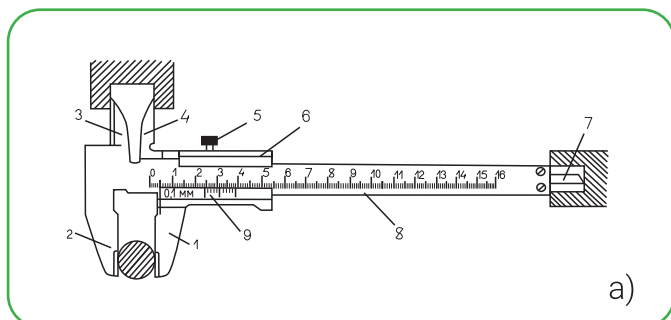
Рисунок 24. Штангенциркуль марки ШЦ-I:
