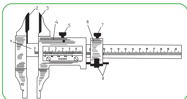
Рисунок 25. Штангенциркуль марки ШЦ-II: 1 – штанга; 2 – неподвижная губка; 3 – подвижная губка; 4 – рама; 5 – винт для фиксации; 6 – хомут; 7 – винт для закрепления хомута; 8 – микрометрический винт.
