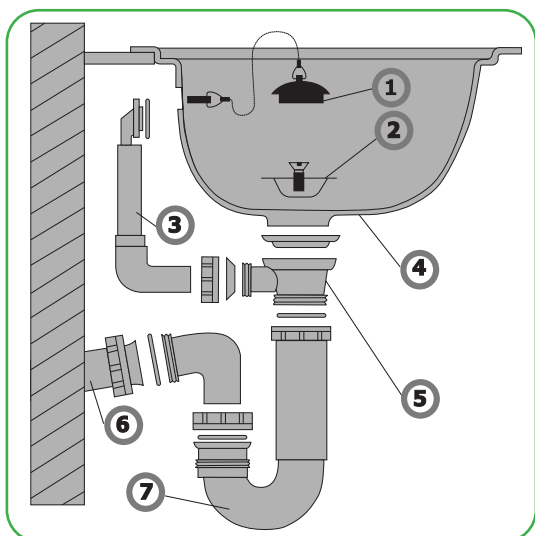
Рисунок 62. Устройства сифона: 1 – заглушка; 2 – болт и сетка; 3 – водоотвод раковины; 4 – раковина; 5 – полость сточной воды; 6 – труба канализационная; 7 – сифон.
