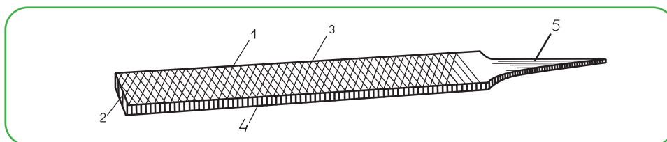
Рисунок 45. Устройство напильника: 1 – рабочая часть; 2 – наконечник; 3 – край; 4 – боковая часть; 5 – хвост.
