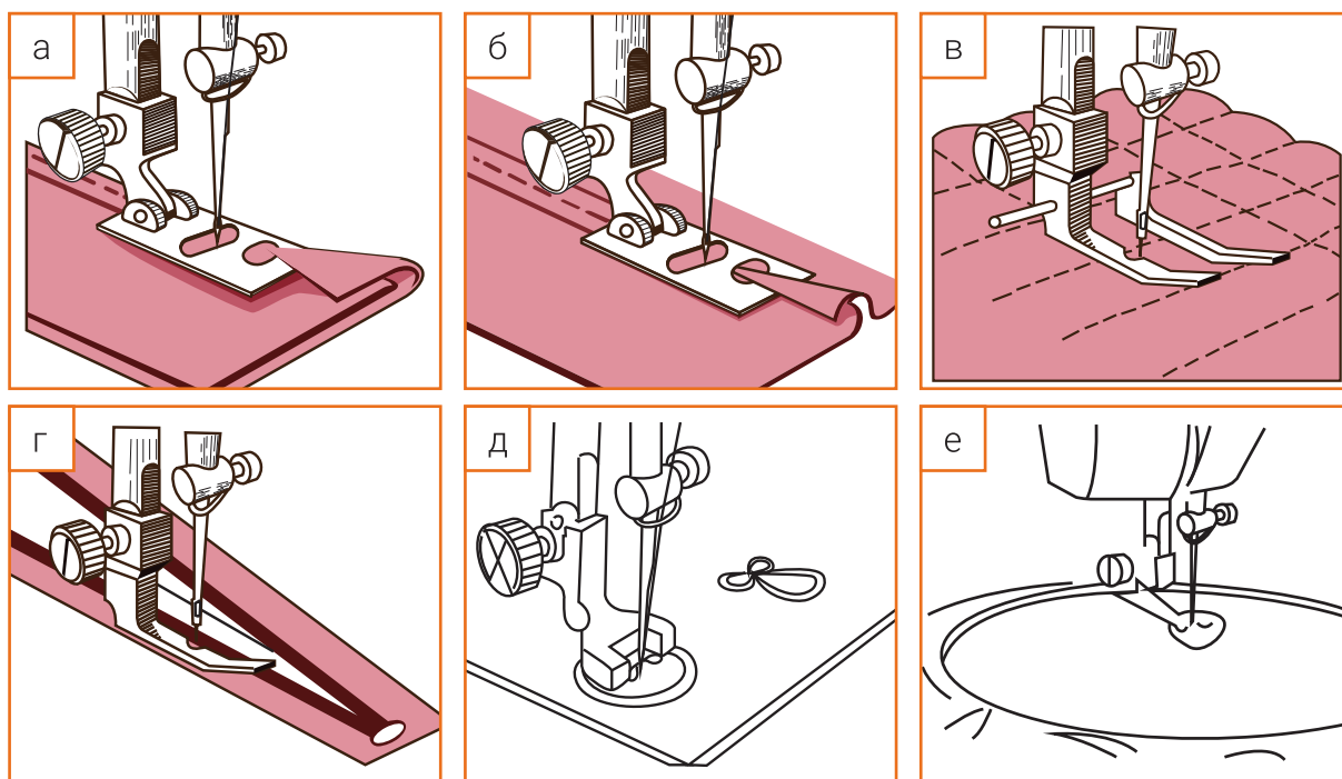
Рисунок 10. Приспособления малой механизации для швейной машинки.
