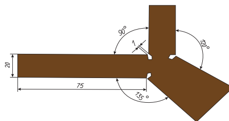
Рисунок 9. Комбинированный угломер.
