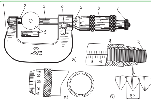
Рисунок 27. Микрометр: а) устройство: 1 – скоба; 2 – пятка; 3 – винт; 4 – стопор; 5 – стержень; 6 – барабан; 7 – трещётка; 8 – стержень; б) микрометрический винт; в) барабан.
