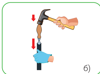
Рисунок 46. Установка ручки напильника: а) установка ручки; б) крепление ручки.
