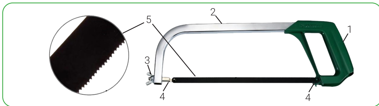
Рисунок 32. Устройство пилы: 1 – ручка; 2 – рама; 3 – стяжной винт и ушко (барашка); 4 – штифты; 5 – полотно (пила).
