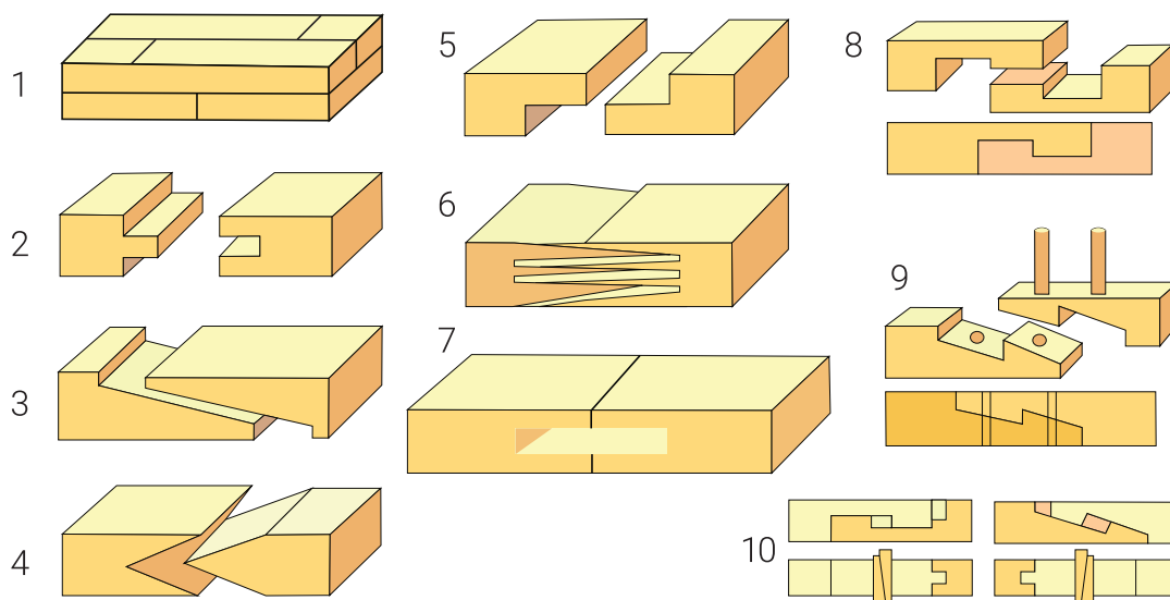
Рисунок 22. Способы сращивания и наращивания: 1 – впритык; 2 – гребёнка; 3 – по прямой; 4 – клиновидный; 5 – с бортиком; 6 – зубчатый; 7 – с вставным клином; 8 – накладной в виде замка; 9 – ступенчатый с шпунтом; 10 – прямой и косой замок.
