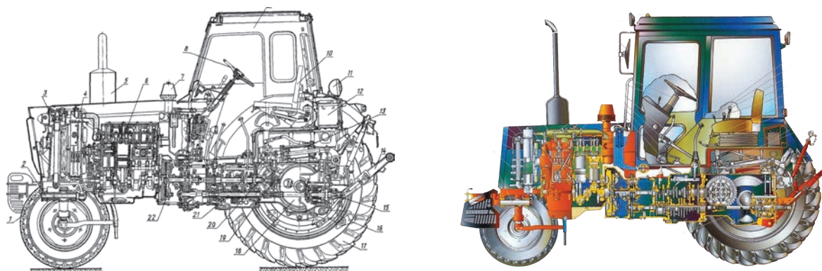
Рисунок 8. Устройство универсально-пропашного трактора МТЗ-80, схема расположения узлов и агрегатов:
