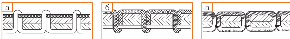
Рис 11. Дефекты машинного шва и правильная строчка:
