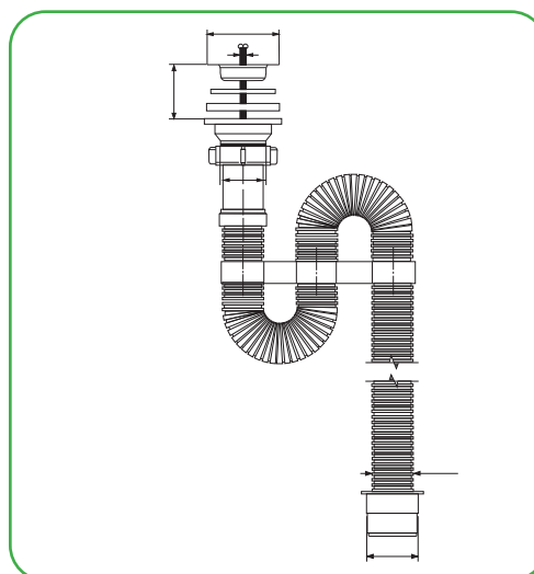
Рисунок 61. Принципиальная схема последовательности сборки гофрированного сифона AC-3011.
