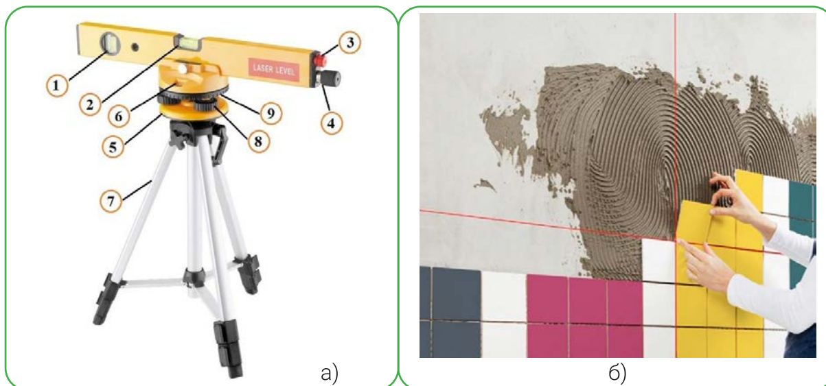
Рисунок 12. Лазерный уровень:
