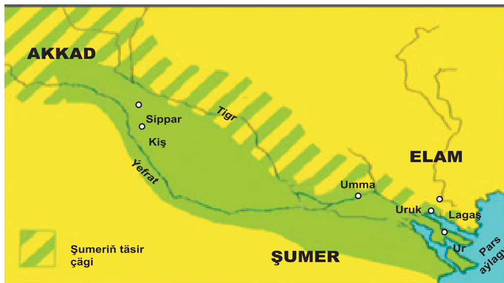
Mesopotamiyanyň kartasy
