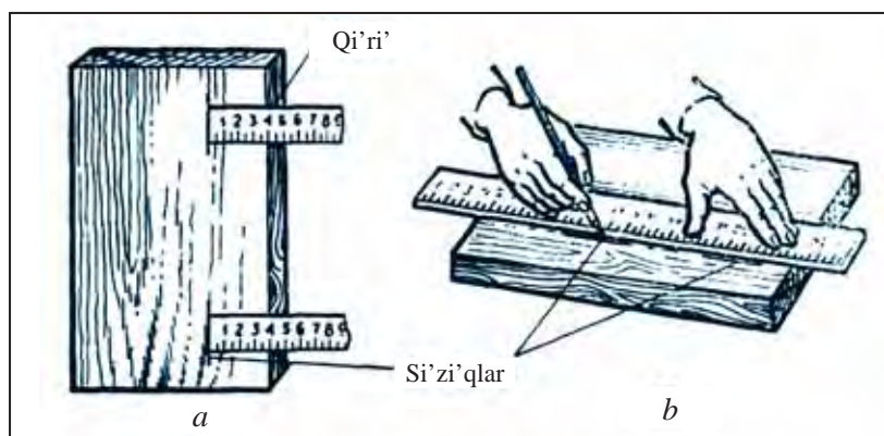
40-su'wret. Masshtabli' si'zg'i'sh ja'rdeminde detaldi' rejelew: a) detaldi'n' yenin wo'lsheiw; b) reje si'zi'g'i'n wo'tkeriw.
