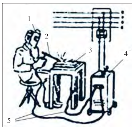
27-su'wret. Elektr kepslerlew ushi'n u'skeneler: 1-qorg'awshi' maska; 2-elektrod; 3-buyi'm; 4-kepslerlew aparati'; 5-si'mlar.
