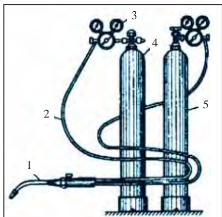
26-su'wret. Gaz benen kepslerew ushi'n u'skeneler: 1-gorelka; 2-shlanglar; 3-reduktor; 4-kislorodli' ballon; 5-acetilenli ballon.
