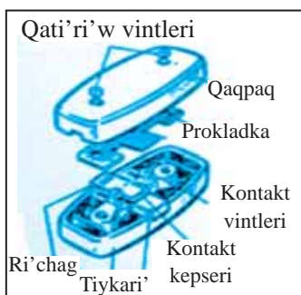
75-su'wret. Aspa aji'ratlari'p-qosqishti'n du'zilisi.
