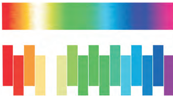
Rangli spektr
