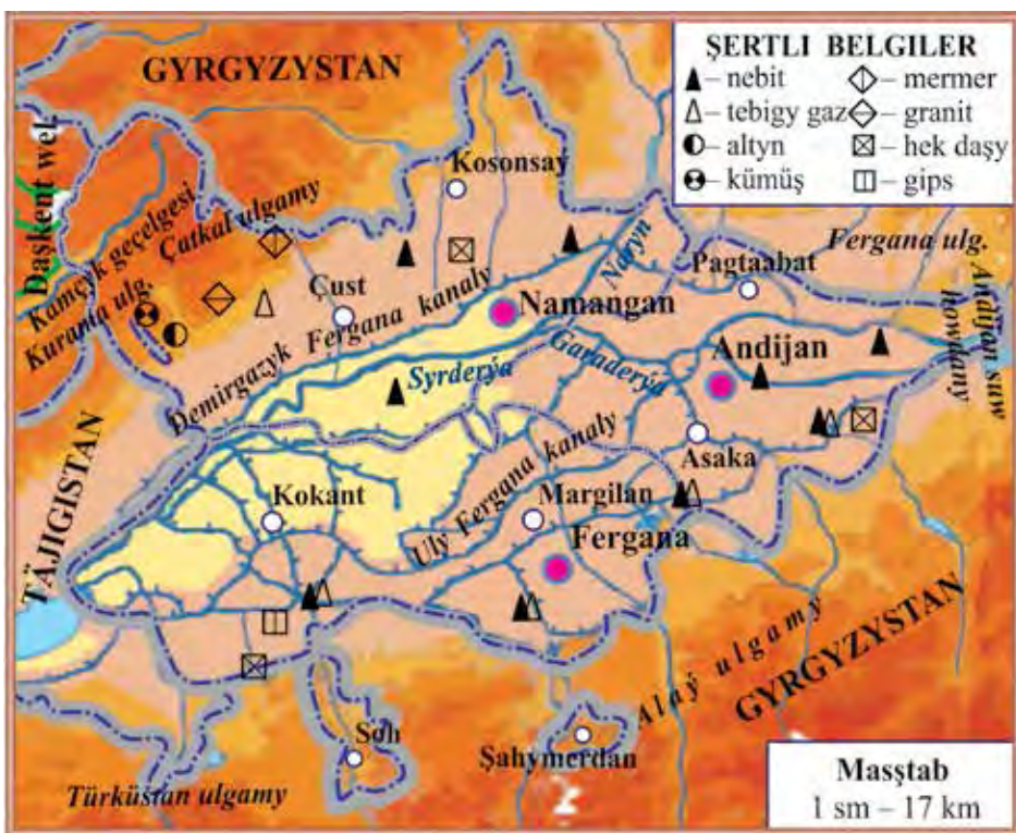
56-njy surat. Fergana jülgesiniň fiziki kartasy.
