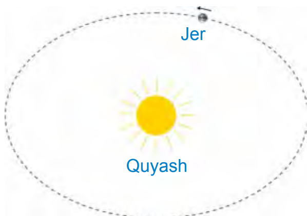
3-súwret. Jer Quyashtırń átirapında aylanadı.
