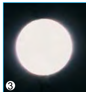
12-súwret. Aydin ozgergen korinislari: 1 – jańa ay; 2 – yarım ay; 3 – tolıq ay.
