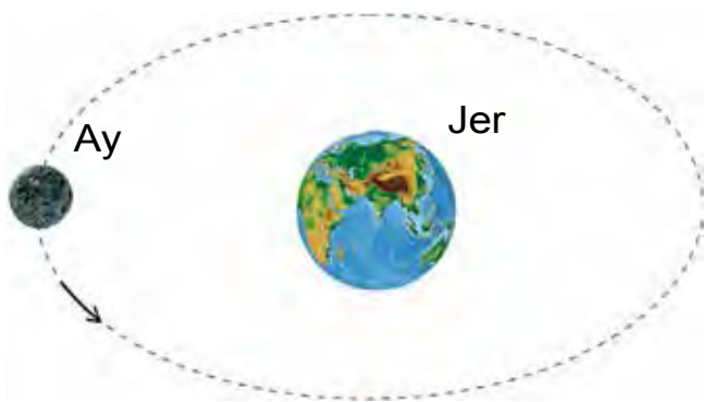
10-súwret. Aydıń Jer átirapında aylanıwı.
