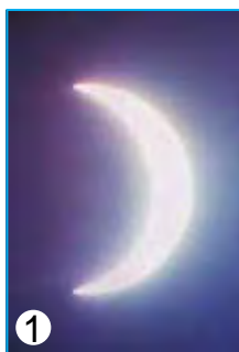
12-súwret. Aydin ozgergen korinislari: 1 – jańa ay; 2 – yarım ay; 3 – tolıq ay.
