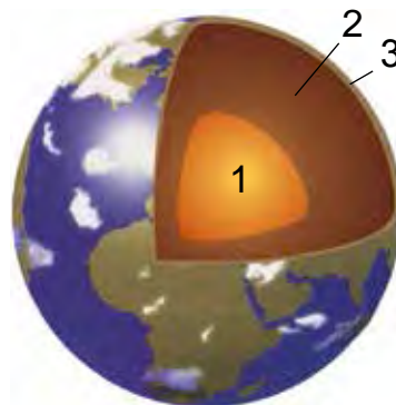
13-súwret. Jer sharınıń ishki dúzilisi.
