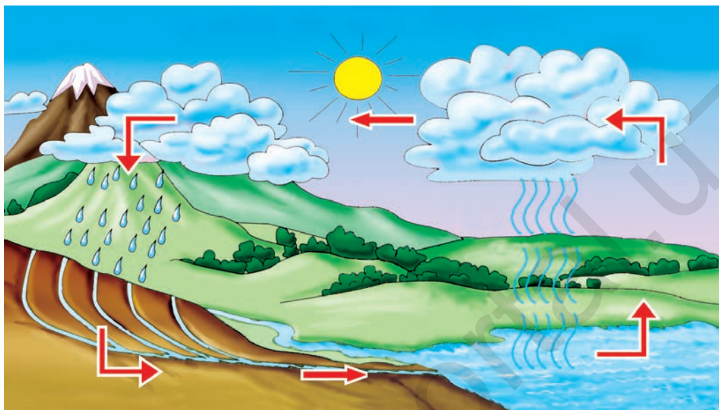
23-súwret. Tábiyattaǵı suwdıń aylanısı.
