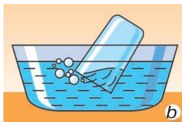
17-súwret. Stakanniń ishinde hawa bar.
