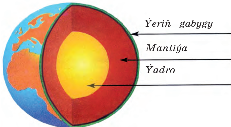
24-nji surat. Ýeriň içki gurluşy
