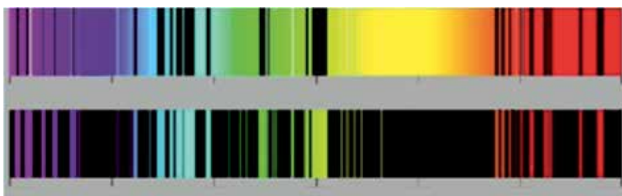
Stronsiy elementining spektri
