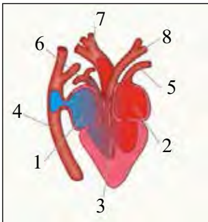
72-сúwret. Jer bawırlawshılardıń dúzilisi; 1-оń бóлме-ше; 2-шеp бóлме-ше; 3-қарınша; 4-gewek vena; 5-óкпе венасы; 6-óкпе артериясы; 7-оń аорта дугасы; 8-шеp аорта дугасы.
