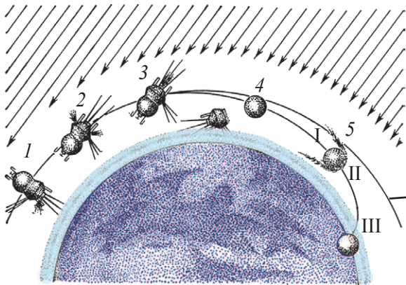
Расми 122. Чараёни аз мадор фаровардани РМ. 1 – 3 импулси тормоздиҳанда; 4 – аз мадори доиравӣ баромадан; 5 – тормози (бозисти) аэродинамикӣ ва бо ёрии парашют фурудой.
