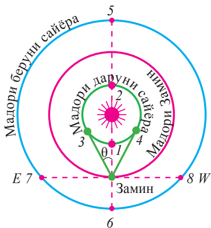
Расми 28. Конфигуратсияи сайёраҳо ва шартӣ намудории онҳо.
