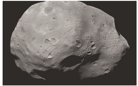
Расми 69. Радифи Марс бо номи Фобос (андозааш 18×22 км).
