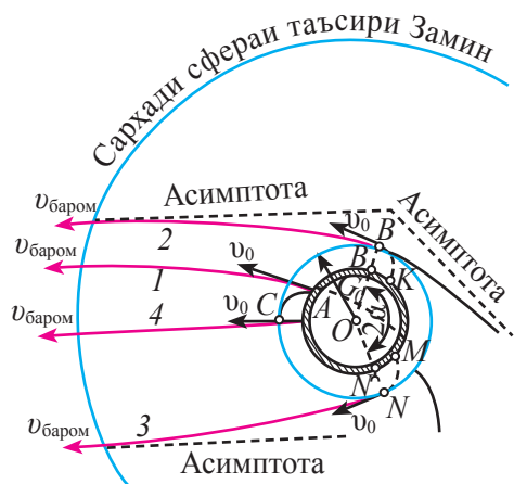
Расми 125. Траекторияҳои имконпазири АК дар сарҳади кураи таъсири Замин барои парвоз ба сайёраҳо (дар ин ҷо 1, 2, 3 ҳо – гиперболӣ, 4 – траекторияи ростхатта аст).
