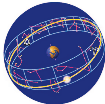
Расми 6. Бурҷҳои ситораҳое, ки дар ҳамвории эклиптика ҷойгир шудаанд—соҳаи зодиаки.
