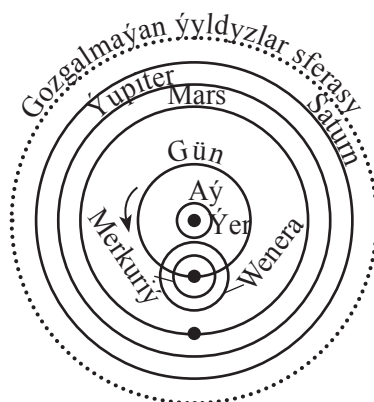
25-nji surat. Birunyň älemiň gurluşy baradaky garaýyşlaryna görä, Gün öz daşynda aýlanýan hemralary – Merkuriý we Wenera bilen bile Ýeriň daşynda aýlanýar.
