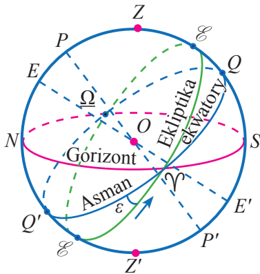
5-nji surat. Günüň ýyllyk görünme hereketi. Ekliptika ( \varepsilon —eklIPTIKA we asman ekwatorynyň emele getiren burçy).
