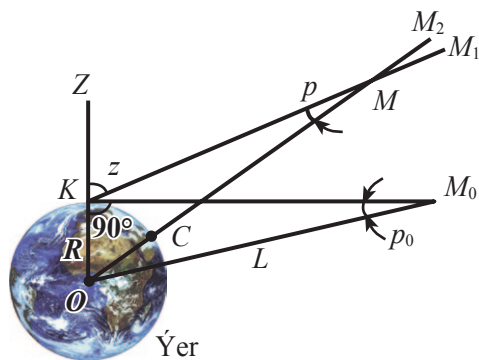
29-njy surat. Ýagtylgyçlaryň sutkalyk ( p ) we sutkalyk gorizont ( p_0 ) parallaksy
