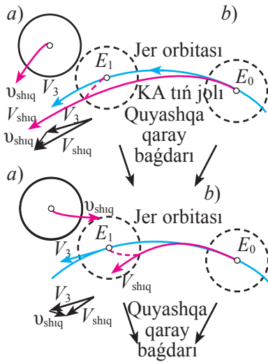
124-súwret. KA tñ Jer tásir sferasındaǵı háreketi: a hám b (joqarıda) – sırtqı planetalarǵa ushıw; a hám b (tómende) – ishki planetalarǵa ushıw sxemaları; a ) geosentrik; b ) geliosentrik traektoriyalar.
