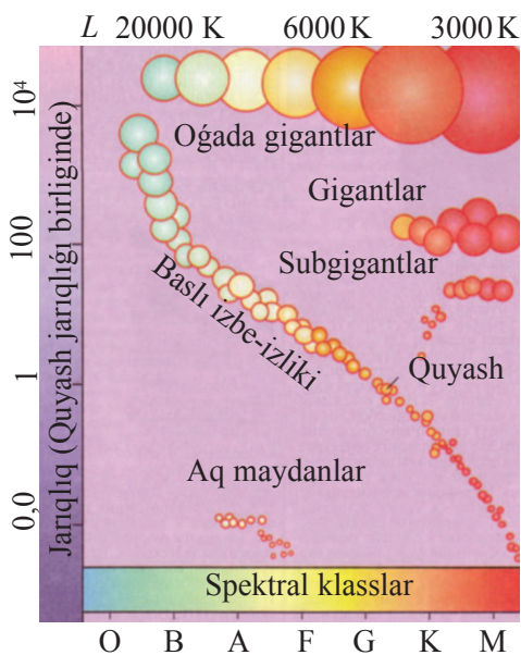
93-súwret. Spektr-jariqlıq diagramması.
