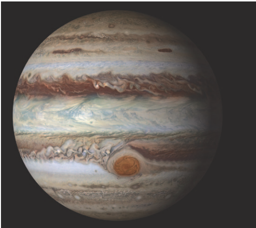
70-súwret. Yupiterdiń ulıwma kórinisi.
