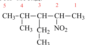
3-этил-4-метил-2-нитропентал
