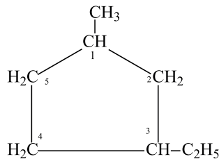
1-метил-3-этилсиклопентан
