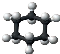
Сиклогексан
