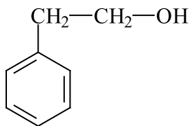
2 - этаноли фенил
