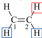
этилен
