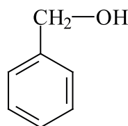
спирти бензил
