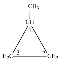
метилциклопропан
