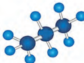
пропан
