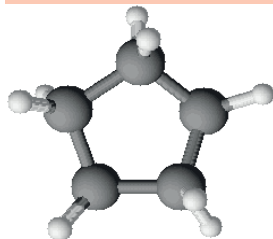
Сиклопентан
