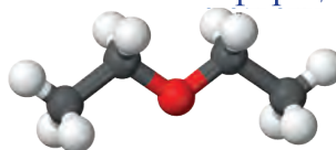
эфири диетил
