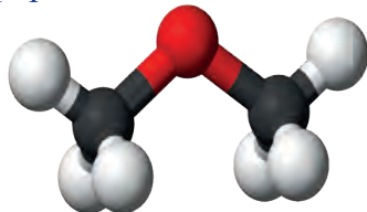
Диметилэфир
