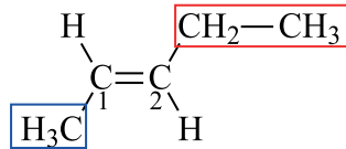
транс-бутен-2
