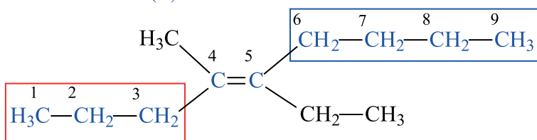
(E)-3-метил-4-этилгептен
