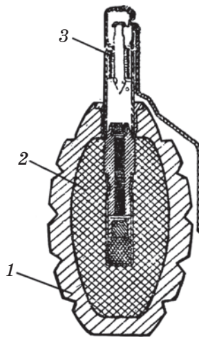
Рис. 116. Устройство ручной осколочной гранаты Ф-1: 1 — корпус; 2 — разрывной заряд; 3 — запал
