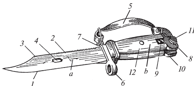
Рис. 103. Штык-нож: a — лезвие; б — рукоятка. 1 — режущая грань; 2 — пила; 3 — заточенная кромка; 4 — отверстие; 5 — ремень; 6 — кольцо; 7 — зацеп для ремня; 8 — металлический наконечник; 9 — соединительный винт; 10 — продольные пазы; 11 — защелка
