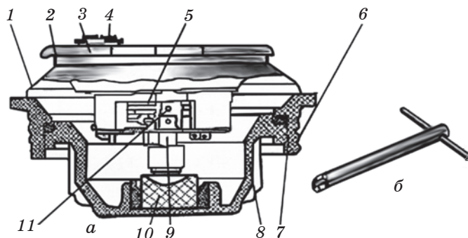
Рис. 78. Взрыватель МВЧ-62:
