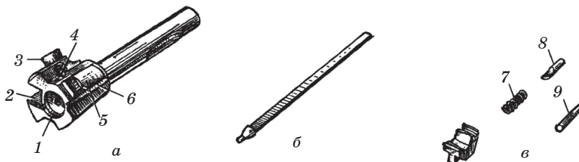
Рис. 97. Затвор: а — остов затвора; б — ударник; в — выбрасыватель.
