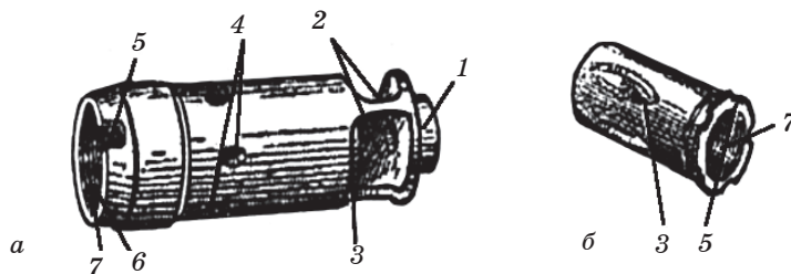
Рис. 92. Дульный тормоз-компенсатор и пламегаситель: a — дульный тормоз-компенсатор; б — пламегаситель. 1 — венчик; 2 — окна; 3 — щель; 4 — компенсационные отверстия; 5 — выем для фиксатора; 6 — скос; 7 — внутренняя резьба
