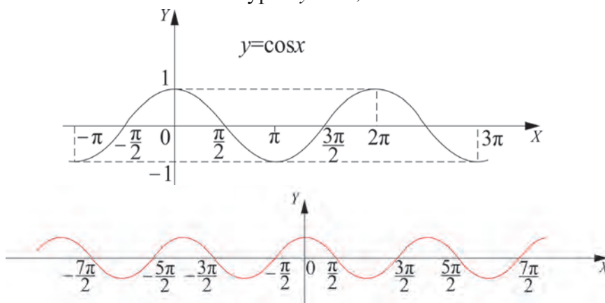
15-сурет. y=\cos x , x \in \mathbb{R} .
