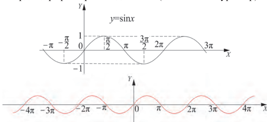
14-сурет. y=\sin x , x \in \mathbb{R} .
