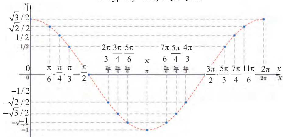
13-сурет. y = \cos x , 0 \leq x \leq 2\pi .
