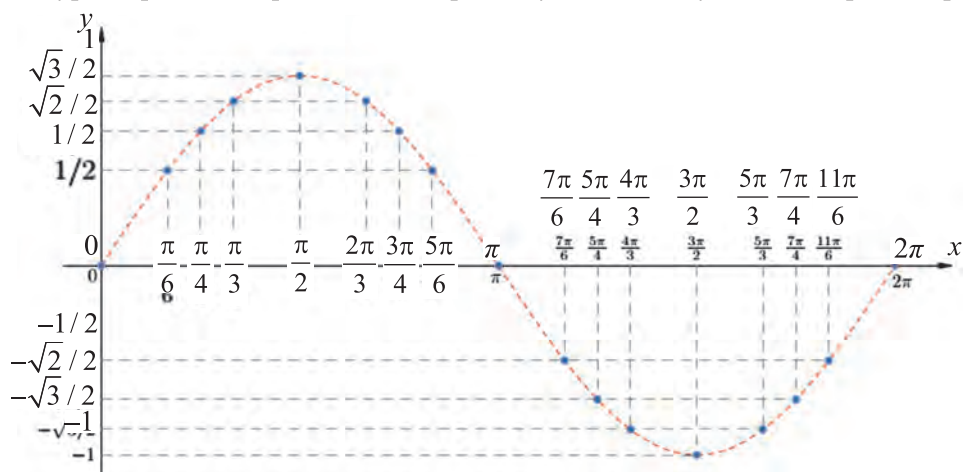
12-сурет. y = \sin x , 0 \leq x \leq 2\pi .
