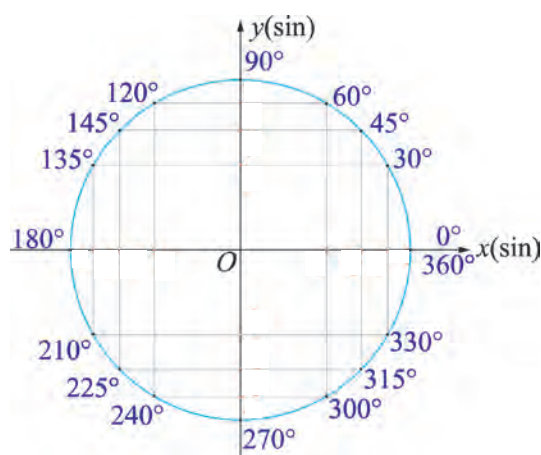
11-сурет. Тригонометриялық шеңбер. Синус пен косинустың кейбір мәндері.
