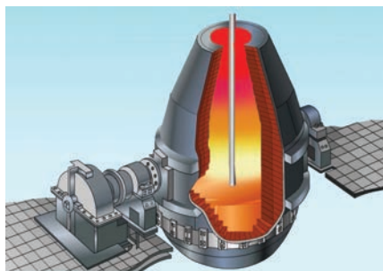
Рис. 19. Кислородный конвертор
