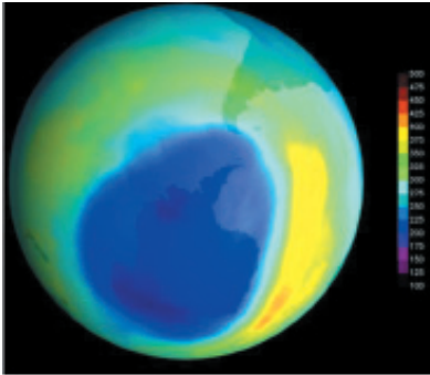
5-súwret. Antarktidanın üstinde ozon qatlami juqalanıwınıń sxemalıq kórinisi.
