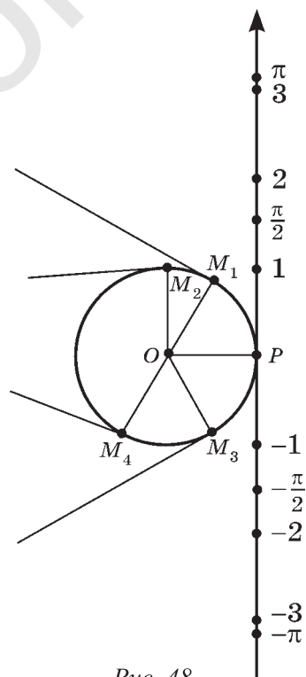
Таким образом, каждой точке прямой ставится в соответствие некоторая точка окружности .
