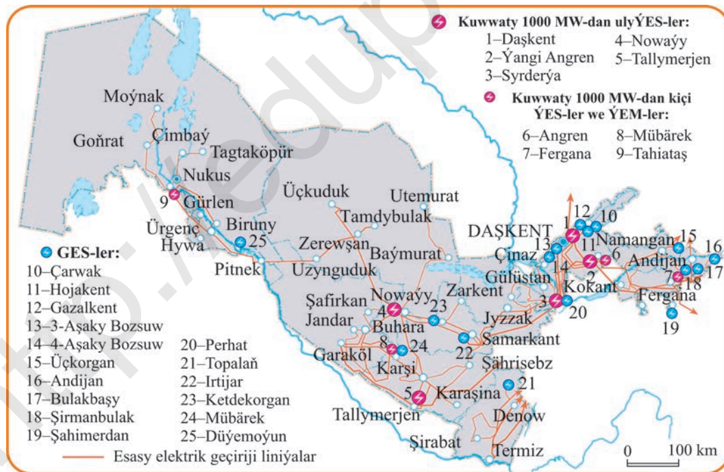
29-njy surat. Özbeğistandaky esasy elektrostansiýalar we elektrik geçiriji liniýalar.
